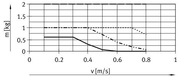
DGSL-10
