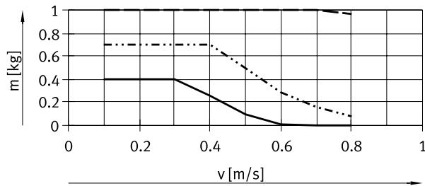
DGSL-8
